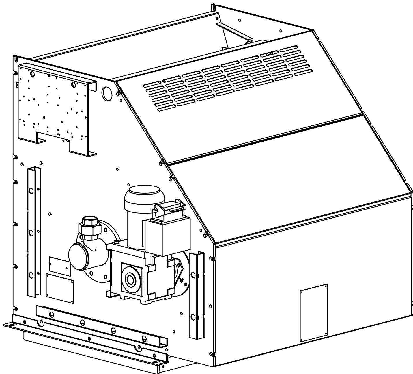
Variante: 75 515 401986 0-0-0-0-0 (Einlauf Rechts; Vliesaufnahme oben)
